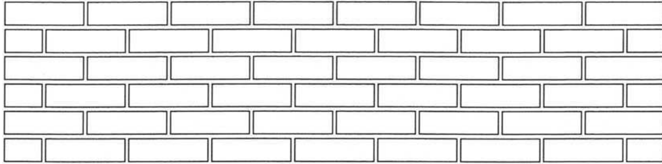
長手積 Strecher bond 210x60xt100/JISサイズ
