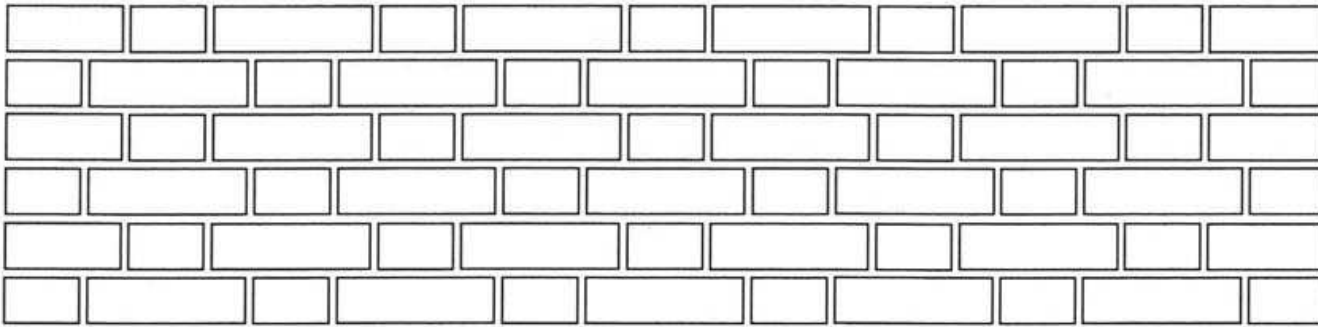
フランス積 Flemish bond 210・100x60xt100
