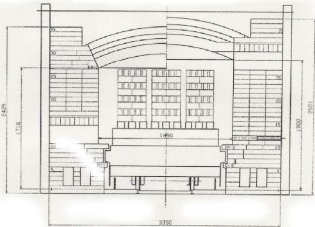
キルン断面図
