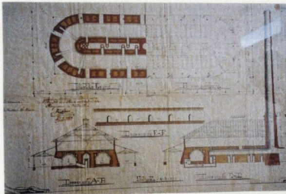
ホフマンキルン（リンクキルン）3つのブロックの単窯
