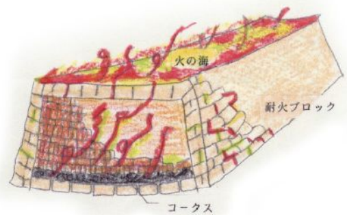
ファイヤーキルン 6週間焼成・150万本生産/回
